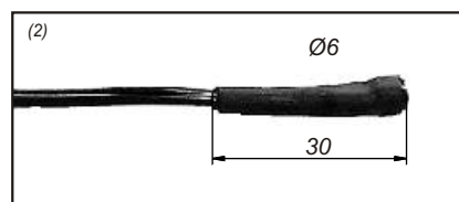
SONDA PTC2000 ECO CÓD: 4.683 Rango: -40°C a 100°C L. Total: 1.5m opcional 3m. Respuesta: a 25°C da 1950 / 1990 Ω Protección: IP67
