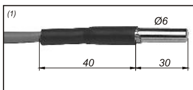
SONDA PTC2000 CÓD: 4.339 Rango: -40°C a 140°C L. Total: 1.5m opcional 3m. (CÓD: 4.343) Respuesta: a 25°C da 1950 / 1990 Ω Protección: IP67
